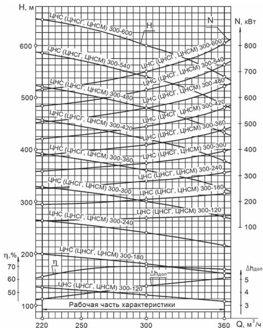
Рис.1.5 Характеристики насосов ЦНС (ЦНСГ, ЦНСМ)300-120...600
