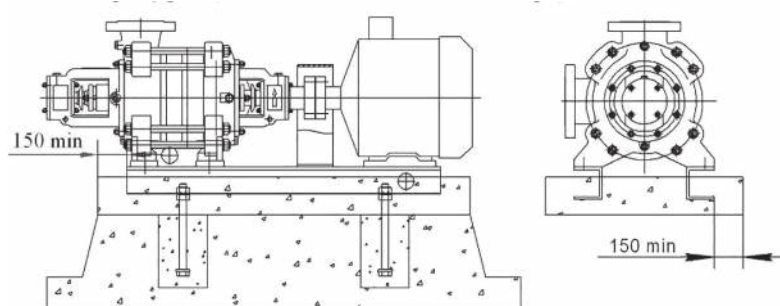
Рисунок 2.2 Установка насоса
