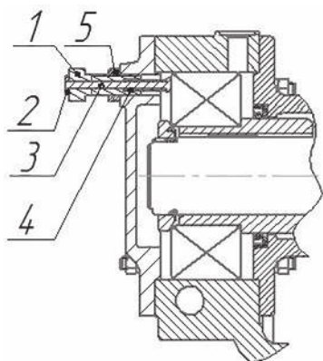
Рис.1.16 Устройство сигнализатора износа гидропаты
