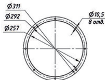
ВЫХОДНОЙ ФЛАНЕЦ
