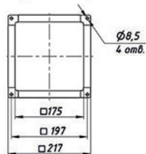
ВЫХОДНОЙ ФЛАНЕЦ
